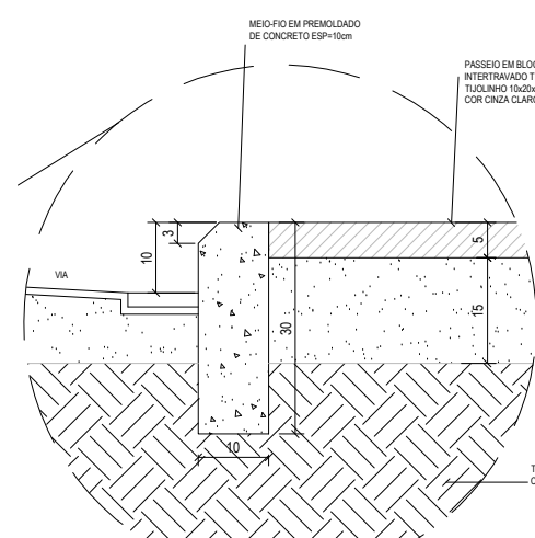
DET. MEIO FIO ESCALA ..... 1:25
