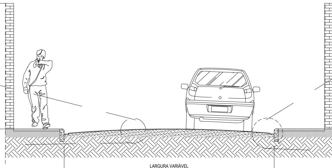
SECÇÃO DA VIA ESCALA ..... 1:50
