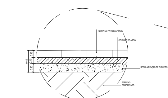
DET. PARALELEPIPADO ESCALA ..... 1:25
