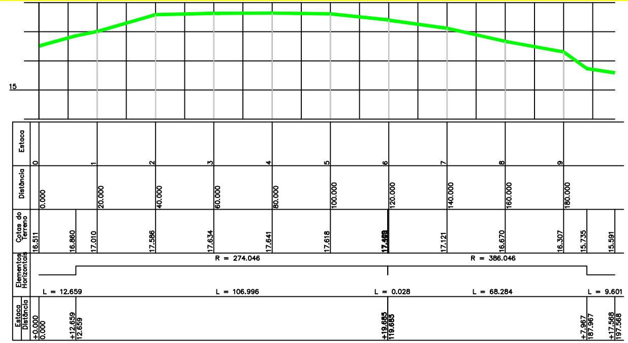
PERFIL LONGITUDINAL ESC: H 1/750 ESC: V 1/75
