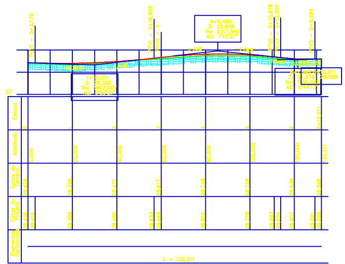
PERFIL LONGITUDINAL ESC: H 1/1000 ESC: V 1/100
