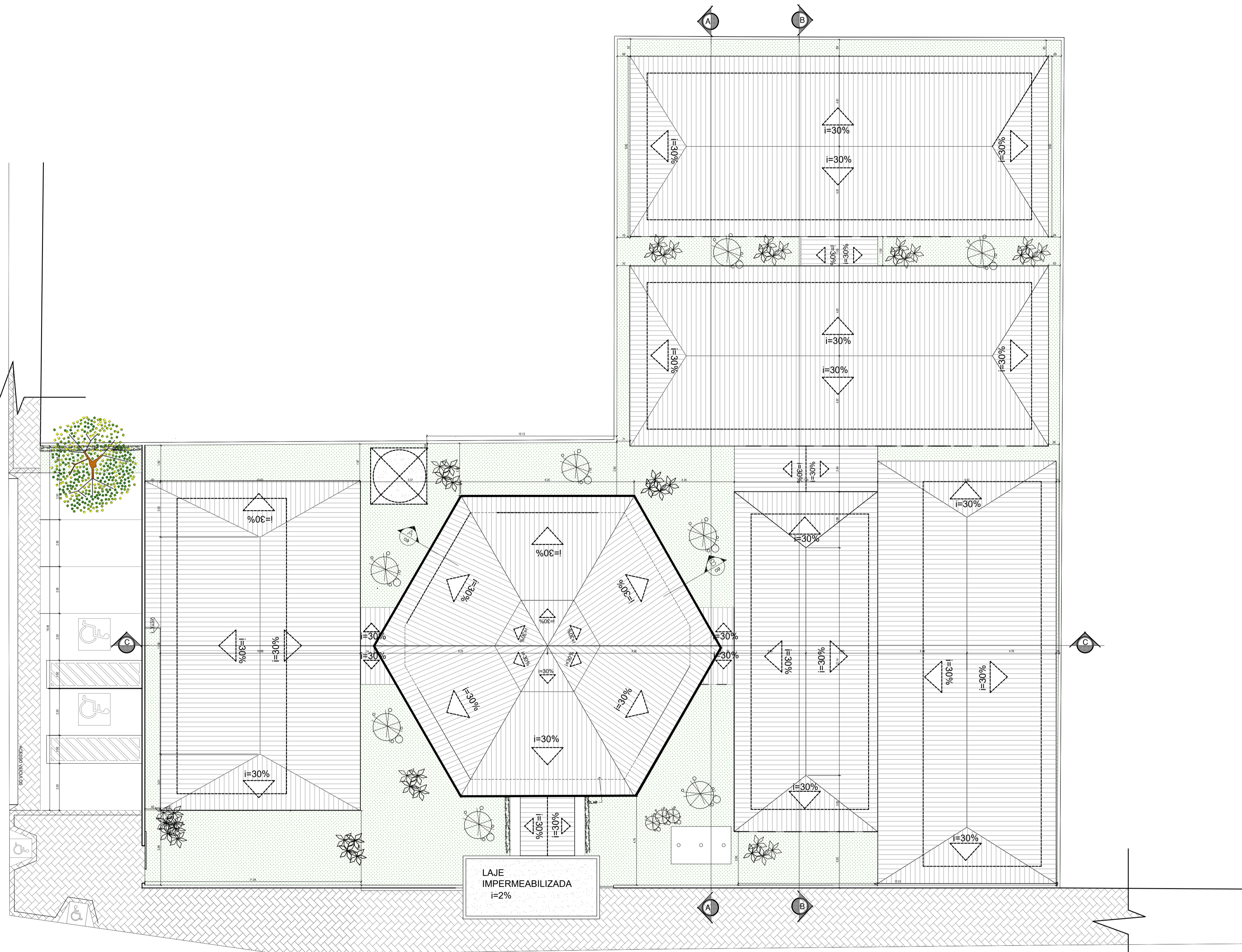
PLANTA DE IMPLANTAÇÃO GERAL BAIRRO DE JARDIM LOLA ESCALA 1/100
